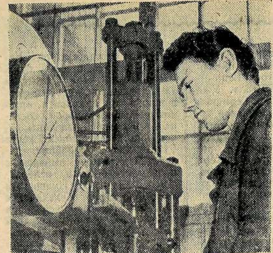
Инженер Г. Ф. Свищев ведёт испытания прочности деталей для подшипников, изготовленных из пластических масс, на первом государственном подшипниковом заводе в Москве. Фото В. Хухлаева.
