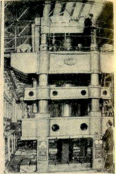
На Рязанском заводе тяжёлого кузнечно-прессового оборудования собран оригинальный гидравлический штамповочный пресс усилием 630 тонн. Он предназначен для холодной штамповки крупных деталей из листового материала. На нем можно производить вытяжные, гибочные и вырезные операции. На снимке: гидравлический штамповочный пресс усилием в 630 тонн. Фото А. Князева.
