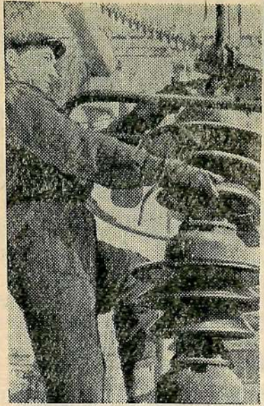
Монтажник Воронежской атомной станции А. Ф. Козочкин регулирует раз'единительное устройство на 220 киловольт. Фото А. Батанова.
