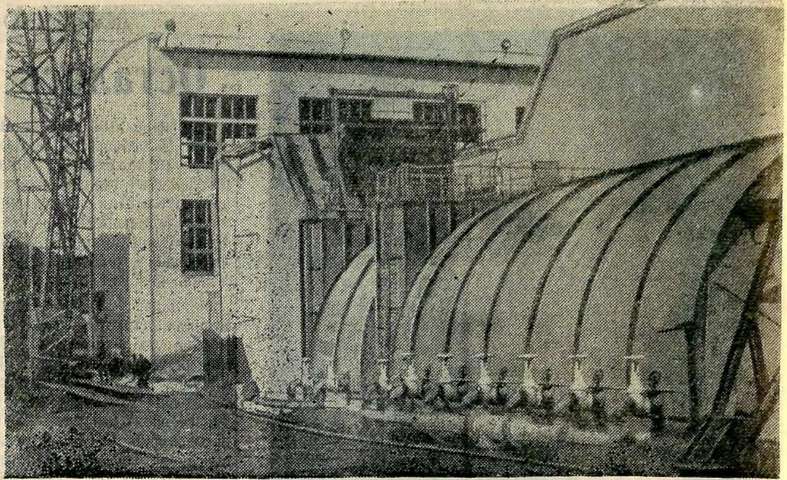
Монтаж газоочистных сооружений комбината искусственного волокна.
