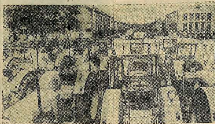
Германская Демократическая Республика. Народный тракторный завод «Нордхаузен» (округ Эрфурт) ежегодно выпускает 6.500 тракторов. Универсальные тракторы «Фамулос-36» и «Фамулос-46» пользуются большим спросом за рубежом. На снимке: тракторы во дворе завода «Нордхаузен» перед отправкой.
