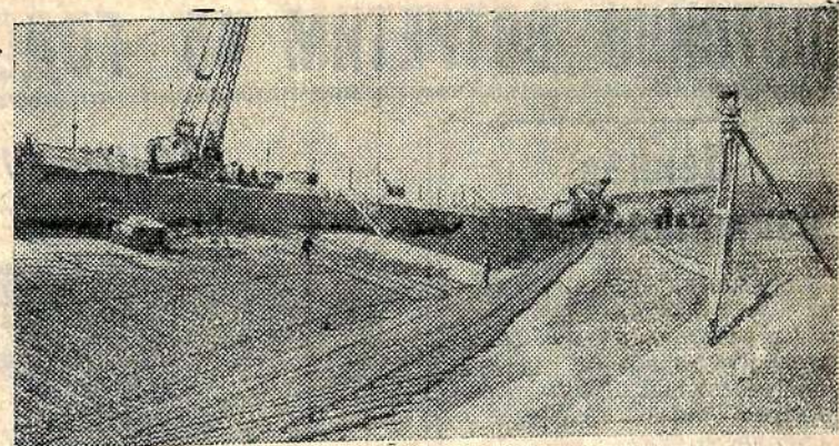
Десятки тысяч кубических метров бетона уложены в фундамент будущего здания Саратовской ГЭС. В настоящее время строители возводят железобетонные плиты водобоя, толщина их 2,5 метра. На снимке: подготовка плиты фундамента здания ГЭС. Фото Е. Соколова.
