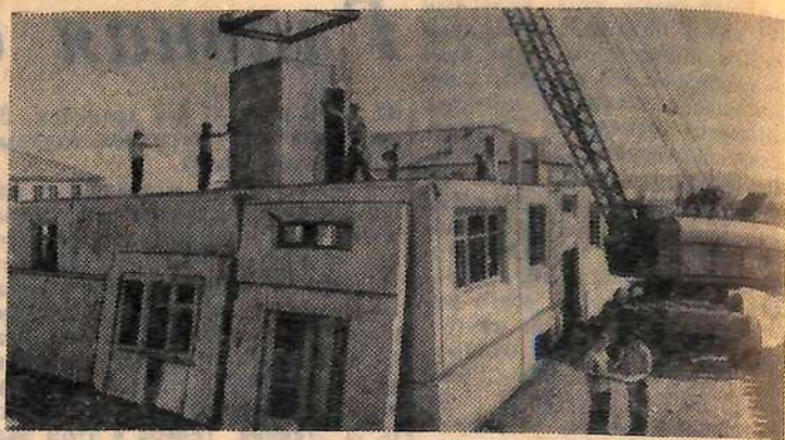
Этот 16-квартирный сборный дом сооружается не в городе, а в селе Менюное, где живут работники Ярославского совхоза (Казахская ССР). Строительство ведет трест "Востокбелсельстрой". Все детали для дома изготовляет коллектив Усть-Каменогорского комбината домостроения. Дома из крупных панелей в сельской местности Восточного Казахстана сооружаются впервые.
