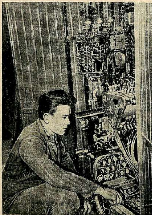
Мастер электроцеха Вольского цементного завода «Красный Октябрь» тов. Соколкин ведет наладку электрофильтра цементных мельниц.
