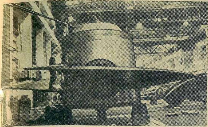
Четвертая турбина мощностью 100 тысяч киловатт для Воткинской ГЭС изготовлена на Металлическом заводе имени XXII съезда КПСС (Ленинград). На снимке: рабочее колесо четвертой турбины. Фото В. Капустина.
