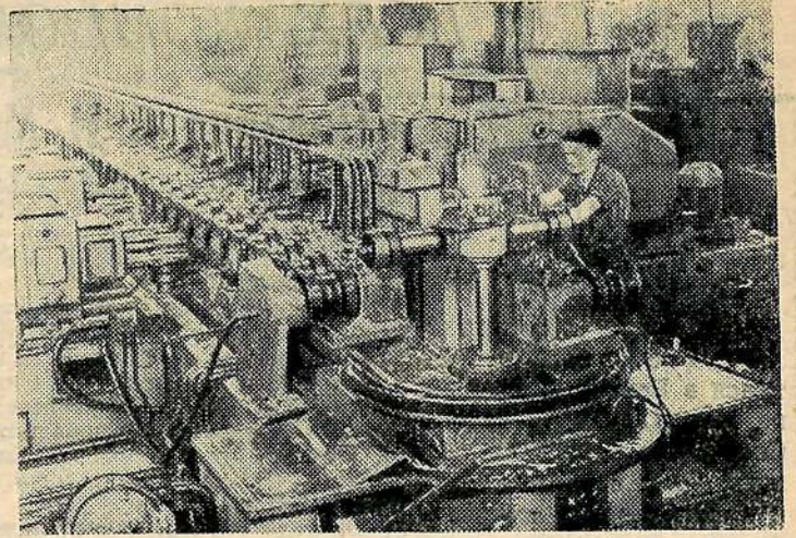
На Челябинском тракторном заводе механизмируются и автоматизируются трудоемкие производственные процессы. Создан ряд автоматических линий, устанавливаются высокопроизводительные агрегатные станки с автоматической подачей деталей. На снимке: автоматическая линия для обработки опорных роликов трактора „С-100“. Линию обслуживают два человека. Раньше на обработке этих деталей было занято 10 человек. Фото Э. Евсерикина.
