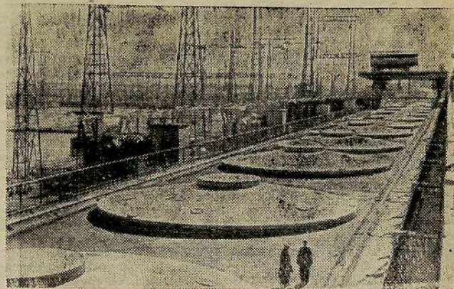
Мощность Кременчугской ГЭС 625 тысяч киловатт. Это станция открытого типа, без здания машинного зала. Она уже вырабатала более 1½ миллиардов киловатт-часов электроэнергии. Фото Г. Верушкина.
