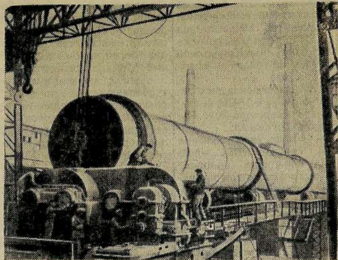
Широким фронтом развернулось строительство второй очереди Кричевского цементно-шиферного комбината (Белорусская ССР). Здесь сооружаются две технологические линии по производству цемента, печное и помольное отделения, другие объекты. Это позволит почти в четыре раза увеличить производство цемента. На 20 дней раньше срока было закончено возведение 100-метровой железобетонной дымовой трубы, досрочно смонтированы три секции корпуса вращающейся печи, раньше графика завершено сооружение ряда других объектов и монтаж технологического оборудования.
