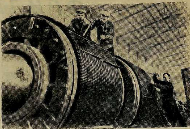
Коллектив харьковского завода „Электротяжмаш“ имени В. И. Ленина заканчивает сборку двух двоярных электрических двигателей общей мощностью 13.200 киловатт для Ждановского металлургического завода имени Ильича.
