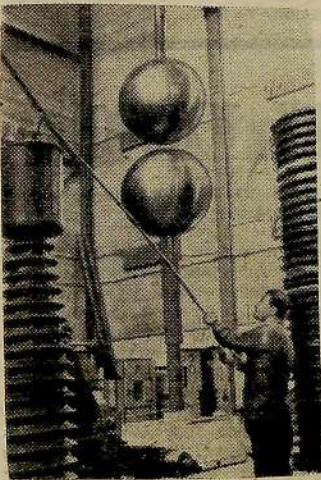
Коллектив московского завода «Изолятор» недавно освоил сложный вид продукции — мощные маслосодержащие вводы напряжением в 220 и 500 киловольт для строительства Братской ГЭС. На заводе успешно выполняются обязательства, взятые по выполнению почетного заказа строителей Братской ГЭС. На снимке: инженер-испытатель Б. П. Ширенков подготавливает ввод на 220 киловольт к электрическим испытаниям. Фото Э. Евзерихина.
