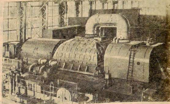
Первый агрегат Назаровской ГРЭС (Красноярский край) дал промышленный ток и вступил в строй действующих. На снимке: турбогенератор № 1 Назаровской ГРЭС мощностью 150 тысяч киловатт.
