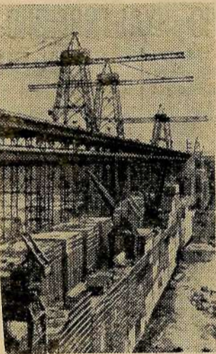
До пуска первого агрегата, который строители Братской ГЭС решили подготовить к открытию XXII съезда КПСС, нужно уложить 700 тысяч кубометров бетона в основное сооружение. На снимке: общий вид плотины с левого берега Ангары. Фото Н. Перка.
