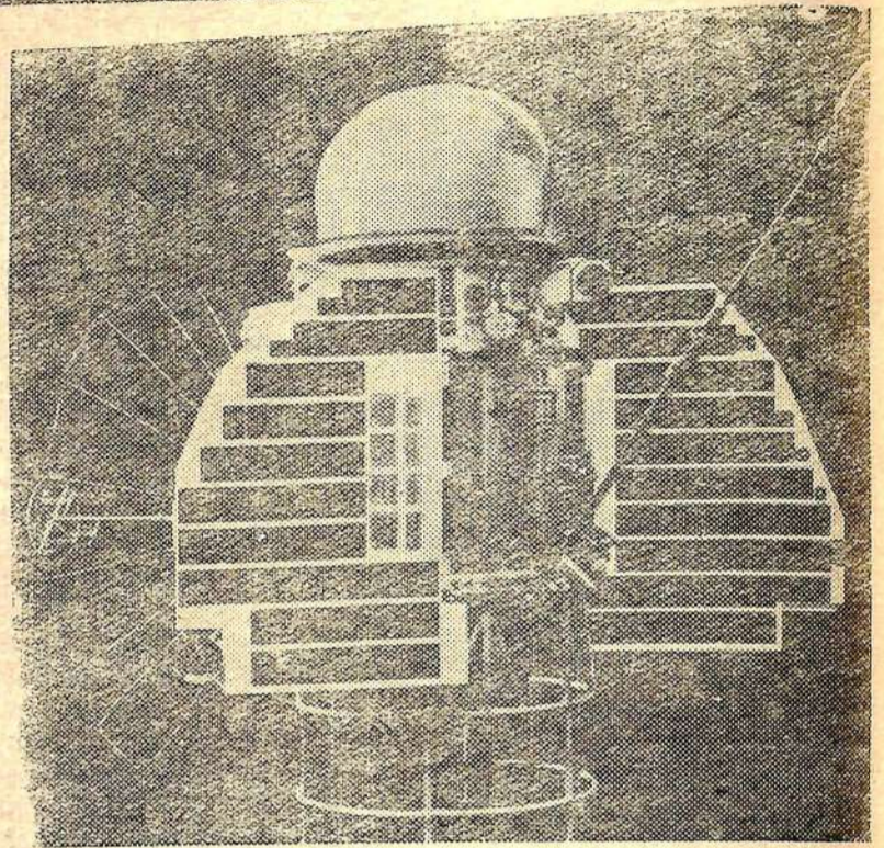
На снимке: автоматическая межпланетная станция на монтажной подставке. Вид спереди. Штыревая антенна установлена в полураскрытом положении.
