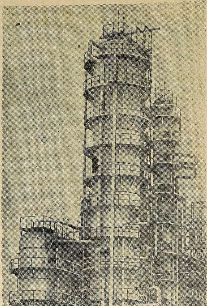
Установка селективной очистки, недавно сланная в эксплуатацию на Сталинградском нефтеперерабатывающем заводе. Фото В. Сметанникова.
