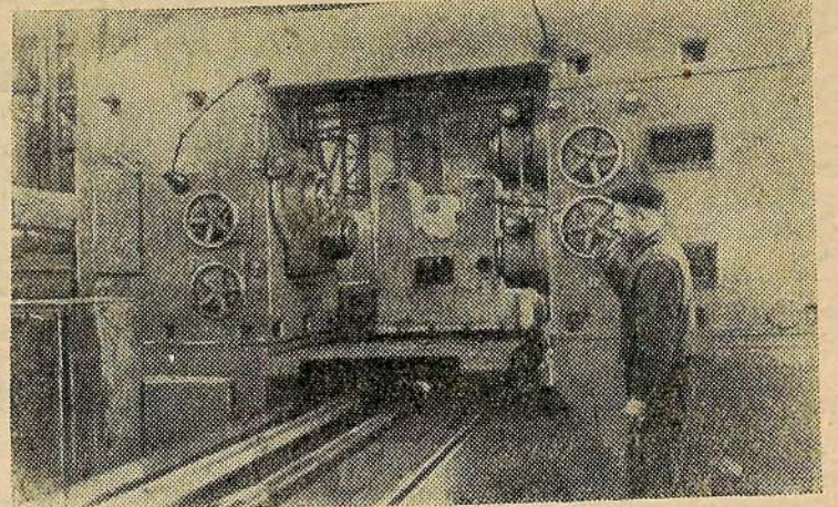
С начала года на ленинградском заводе имени Свердлова создано более 90 уникальных расточных и фрезерных станков. Недавно свердловцы изготовили фрезерный полуавтомат, предназначенный для обработки корпусов двигателей электро-ов. На снимке: бригадир слесарей-сборщиков А. П. Монохов испытывает новый станок.
