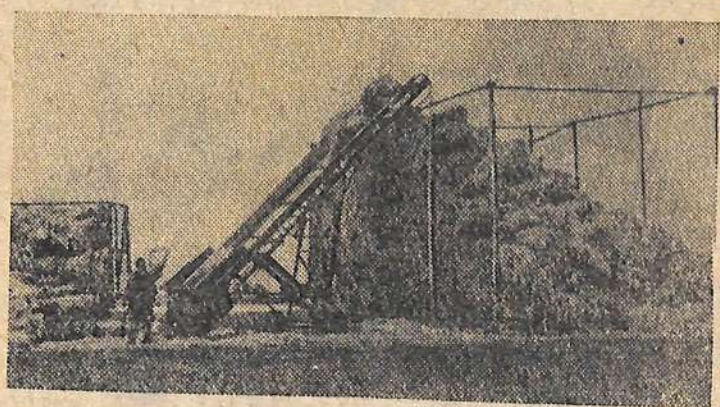
Портативный полевой амбар для хранения сена предложил экспериментальный институт сельскохозяйственных машин в Клузденко (Польша). Емкость контейнера со стенками из проволоочной сетки — 50 тонн.
