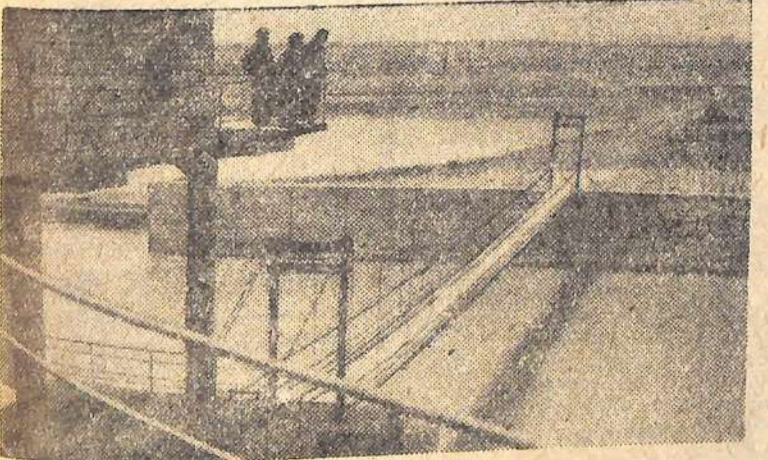
АРМЯНСКАЯ ССР. На строительстве крупнейшей в республике Мхчанской насосной станции идет прокладка и монтаж трехлинейного трубопровода, сооружаются дамбы на Севджурском головном участке и у Нижне-Разданского участка. С вводом станции в эксплуатацию свыше 20 тысяч гектаров земель будет орошаться.
