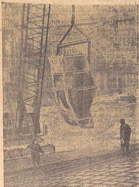
Левобережный верховой ковш гидростанции. Крепление откосов ковша поручено коллективу первого участка восьмого строительного управления. Выполнено больше половины объема гидротехнических работ. Только в январе бригады Волохова и Белянского, несмотря на плохие погодные условия, уложили в сооружение 1400 кубометров бетона. На снимке: рабочие бригады Н. Белянского принимают бетон в карту ковша. Фото М. Бабенко.
