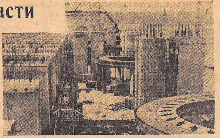
Пусковые секции гидростанции. Третий ярус. Идет монтаж гидросилового оборудования. Фото А. Лекарева.
