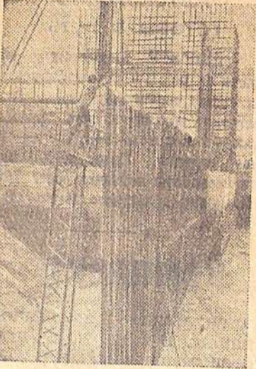
Всего 25 месяцев отделяют нас от того момента, когда волжские воды потекут через агрегаты ГЭС. Сейчас ведется монтаж здания. На этом снимке вы видите, как производится забивка шпунта левого бережной части здания гидроэлектростанции.
