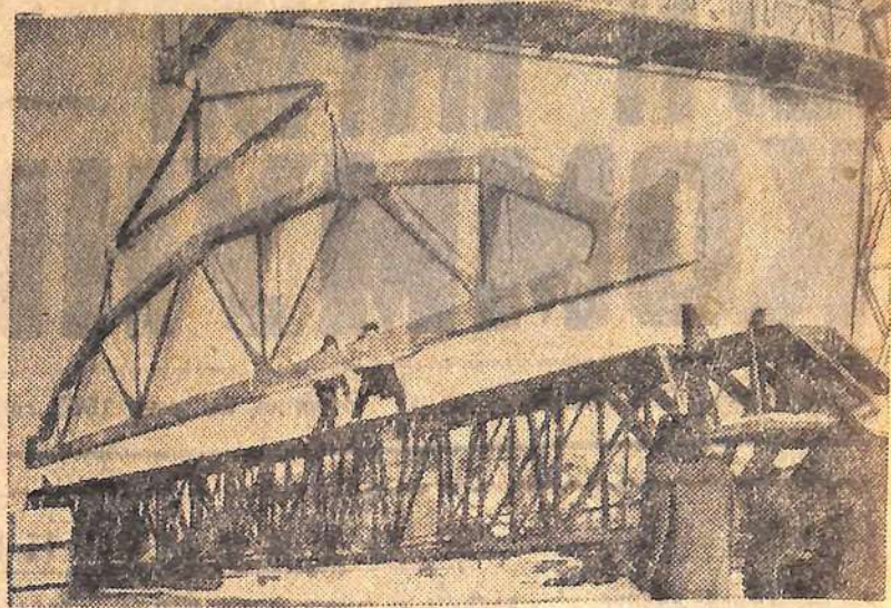
Челябинск. На заводе железобетонных изделий строительного треста № 42 организовано производство железобетонных ферм с пролетом в 24 метра. Фермы армированы прядями из металла с предварительным их напряжением.
