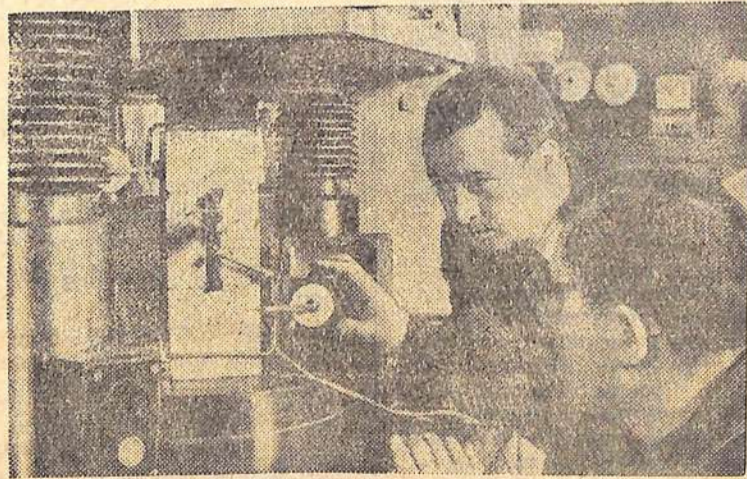
Владивосток. В лаборатории строительных материалов Дальневосточного политехнического института проводятся исследования некоторых видов горных пород Дальнего Востока. Цель этих исследований — получить бесцементные строительные материалы. Опытные образцы высокопрочных вяжущих веществ и бетонов из горных пород Камчатки и Приморья по своим свойствам не уступают лучшим цементным бетонам. Это открывает возможность уже в ближайшее время создать на Камчатке местную промышленность строительных материалов.
