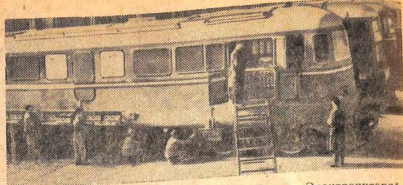
Румынская Народная Республика. Завод «Электропутера» в Крайове выпускает тепловозы мощностью 2.100 лошадиных сил. Из цехов предприятия вышли первые десятки тепловозов такого типа. На снимке: в сборочном цехе завода. Фото Аджерпресс—ТАСС.
