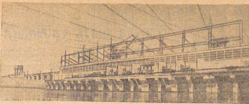
Воткинская ГЭС уже выработала более 1 миллиарда 780 миллионов киловатт-часов электроэнергии. Эта электростанция, строящаяся на Каме, скоро будет пущена на полную мощность. Строители и монтажники соревнуются за сдачу гидроузла правительственной комиссии на год раньше срока. На снимке: общий вид строящейся Воткинской ГЭС. Фото Е. Загуляева.
