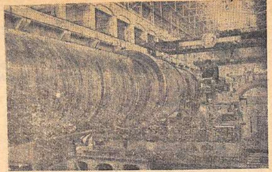
Коллектив харьковских турбо-строителей выполнит почетный заказ: изготовляет для новой стройки на Днепре—Киевской ГЭС горизонтально-капсульные гидротурбины. Эти необычные машины, разработанные конструкторами предприятия, по своим размерам и внешнему виду напоминают ракеты. На снимке: обработка вала капсульной гидротурбины. Вес этой гигантской детали более 40 тонн, а длина 8 метров. Фото Е. Андреева.
