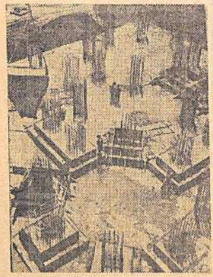
Армянская ССР. В городе Раздане началось строительство крупного цементного завода. На снимке: закладка фундаментов горизонтальных и отвесных известковых бассейнов.
