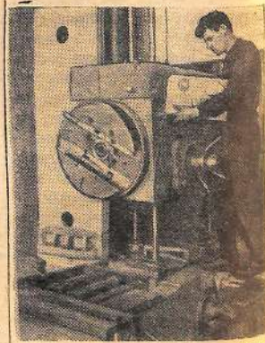
Ленинградский завод имени Свердлова выпускает металлообрабатывающие станки высокого класса точности. Они вытеснили добрую славу не только в нашей стране, но и за рубежом. На сборочных стендах сейчас можно видеть станки, изготовляемые для Китая, Индии и других стран. На снимке: один из станков, изготовляемых заводом. Фото В. Капустина.
