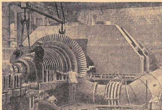
Гигантская паровая турбина мощностью 300 тысяч киловатт, сборка которой показана на снимке, изготовлена Ленинградским Металлическим заводом имени XXII съезда КПСС. Это первая машина для строящейся Коляновской тепловой электростанции, которая будет давать ток системам Мосэнерго и Ленинэнерго. Фото В. Капустина. Фотохроника ТАСС.
