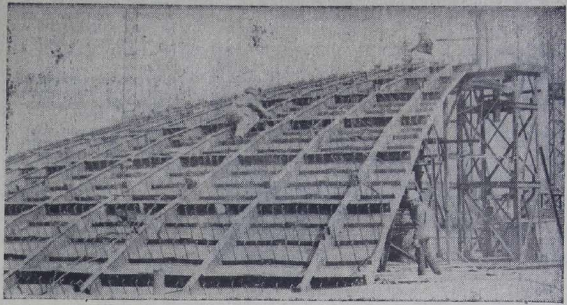
Коллектив бригады монтажников Волжского участка «Гидромонтаж», которым руководит В. Н. Немов, успешно проводит сборку металлоконструкций купола реактора на АЭС.
