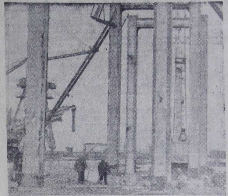
Успешно ведет монтаж сборных железобетонных и металлоконструкций технологической эстакады трубопроводов, которая соединит спецкорпус с реакторным отделением АЭС, коллектив бригады пятого участка Химстроя, руководимый С. В. Калибердой. НА СНИМКЕ: установка опор эстакады. Фото М. Бабенко.
