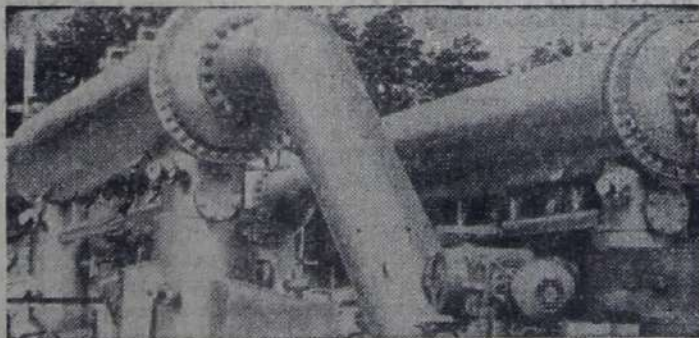
ЧССР. В Пршиборе (Северная Моравия) завершается строительство подземного хранилища газа.
