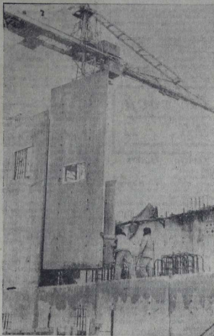
Успешно трудится на монтаже лицевой опалубки первого реакторного отделения атомной электростанции коллектив бригады Героя Социалистического Труда Н. П. Деркача. НА СНИМКЕ: установка элементов опалубки.
