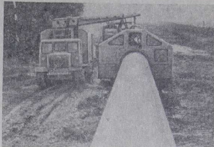
Украинская ССР. На трассе экспортного газопровода Уренгой-Ужгород, проходящего через центральные области Украины, сварены уже десятки километров труб. Всего коллективом специального управления № 12 и строительно-монтажного управления № 10 треста «Укртрубопроводстрой» предстоит проложить 117 километров трассы. Строители включились в социалистическое соревнование по принципу «рабочей эстафеты» за досрочное сооружение трансконтинентальной магистрали.
