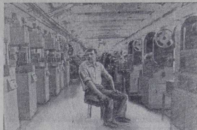
Целое семейство промышленных манипуляторов действует в прессовом цехе Орловского производственного объединения «Промприбор». Внедрение автоматки позволило часть рабочих перевести в другие цеха. Теперь на участке роботов трудится один человек — наладчик. На снимке: наладчик участка промышленных манипуляторов Михаил Докукин. Фото В. Углика (Фотохроника ТАСС)
