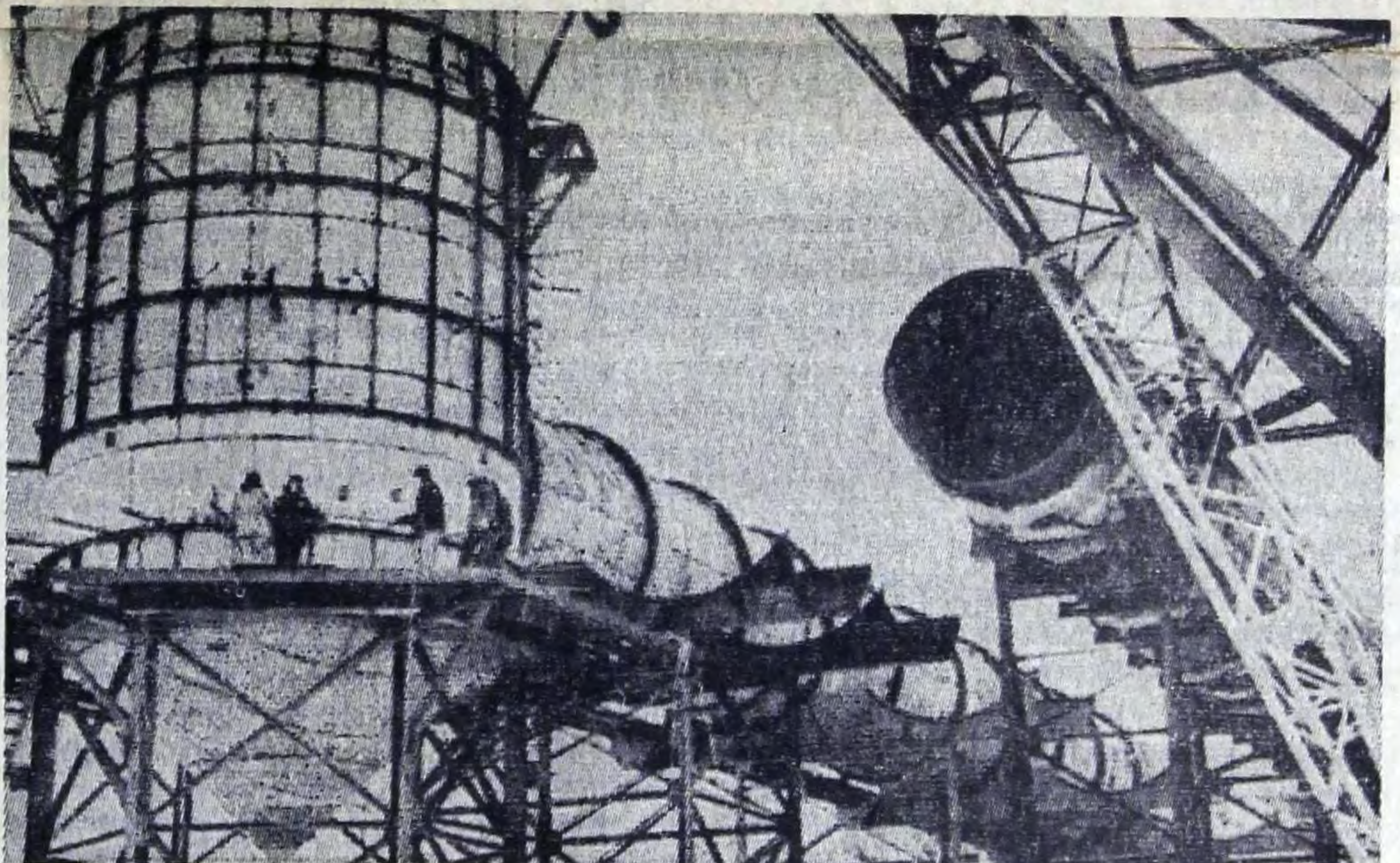
На снимке: монтаж газохода 200-метровой выхлопной трубы. Фото М. Бабенко.
