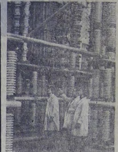
Тольятти. Мощный испытательный стенд для отработки и проверки преобразовательного оборудования, предназначенного для первой в стране линии электропередачи постоянного тока «Экибастуз-Центр», начал действовать в отделении Всесоюзного электротехнического института имени Ленина.
