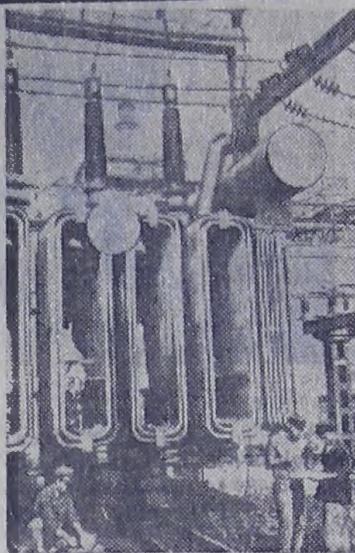
ДРВ. На ТЭС Тхай Нгуен в провинции Бакхай на месяц раньше установленного срока закончен ремонт крупного трансформатора, поврежденного во время бомбардировок американской авиацией. На снимке: восстановленный трансформатор на ТЭС Тхай Нгуен.
