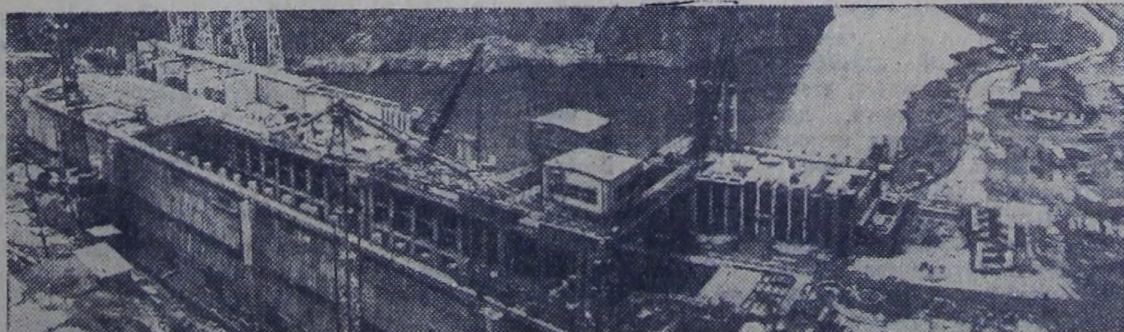
Таджикская ССР. На Вахше, в Пулисангинском ущелье сооружается одна из крупнейших в стране Нурекская ГЭС. 11,2 млрд. киловатт-часов дешевой электроэнергии ежегодно будет давать она промышленным предприятиям и хозяйствам республики. Сейчас на стройке возводится здание ГЭС, монтируются агрегаты, насыпается плотина, высота которой достигнет 300 метров. На снимке: панорама строительства Нурекской ГЭС. Фото А. Кузрина (Фотохроника ТАСС)
