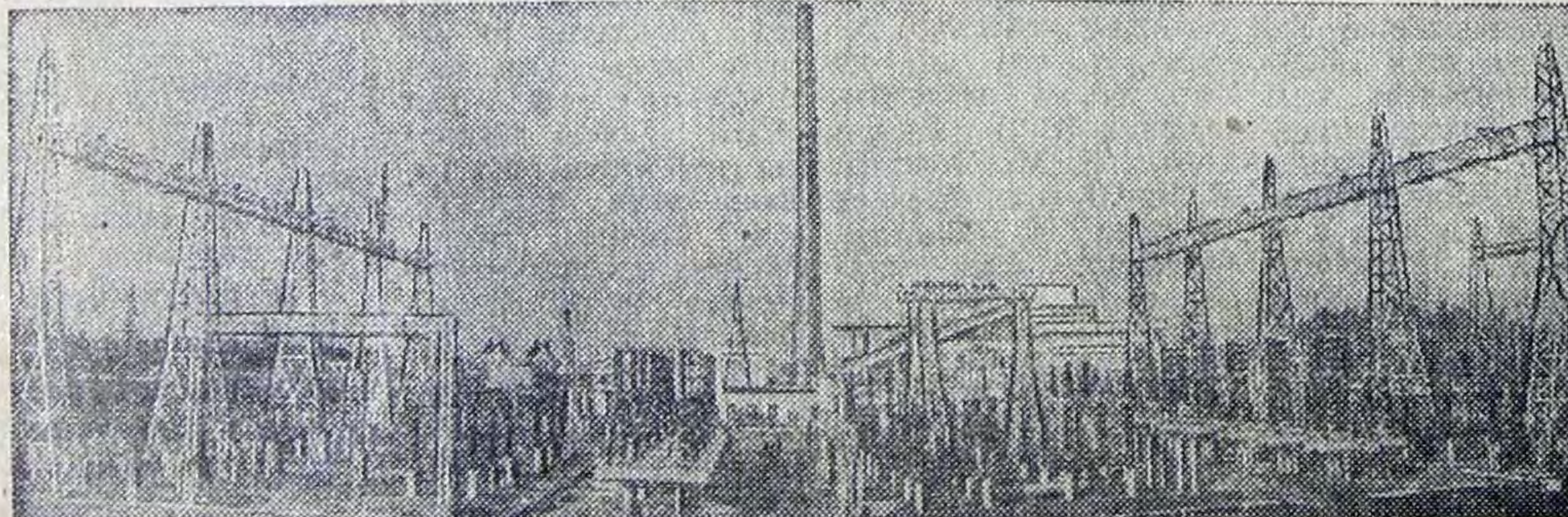
ВИНИЦКАЯ ОБЛАСТЬ. Успешно несет трудовую вахту в честь XXIV съезда КПСС много-тысячный коллектив строителей и энергетиков Ладзынской ГРЭС. На снимке: общий вид открытой распределительной установки Ладзынской ГРЭС. Вдали виден главный корпус станции. Фото Е. Копыта. Фотохроника ТАСС.
