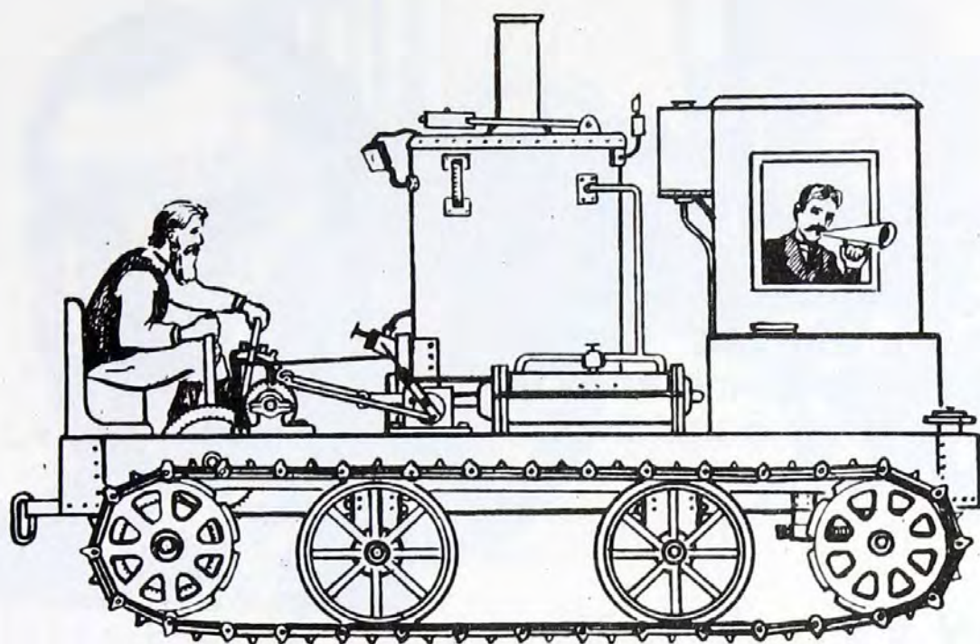
Вторая модификация гусеничного трактора Ф.А.Блинова. Реконструкция проекта автора книги.
